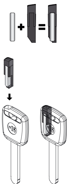
Insert cap / Con tappo a inserimento Glass transponder chip. Transponder in vetro.
