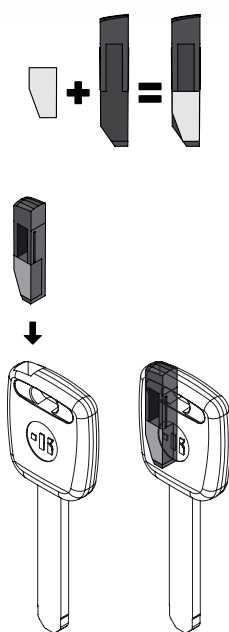
Insert cap / Con tappo a inserimento Carbon transponder chip. Transponder in ceramica.
